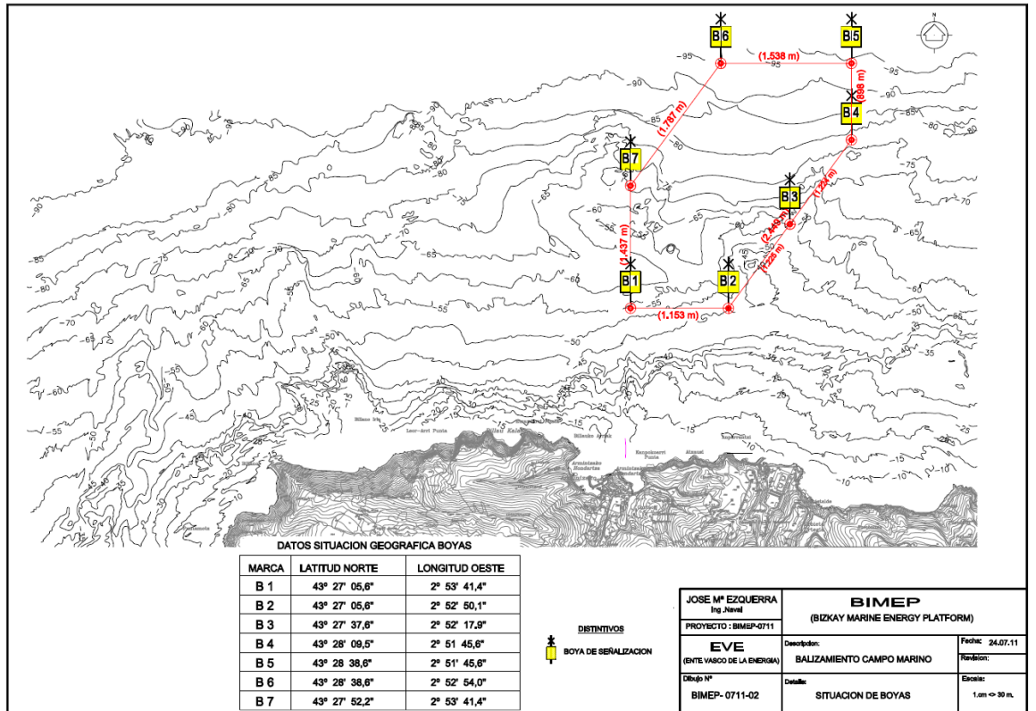
Figura 2 Disposición de las boyas de balizamiento
