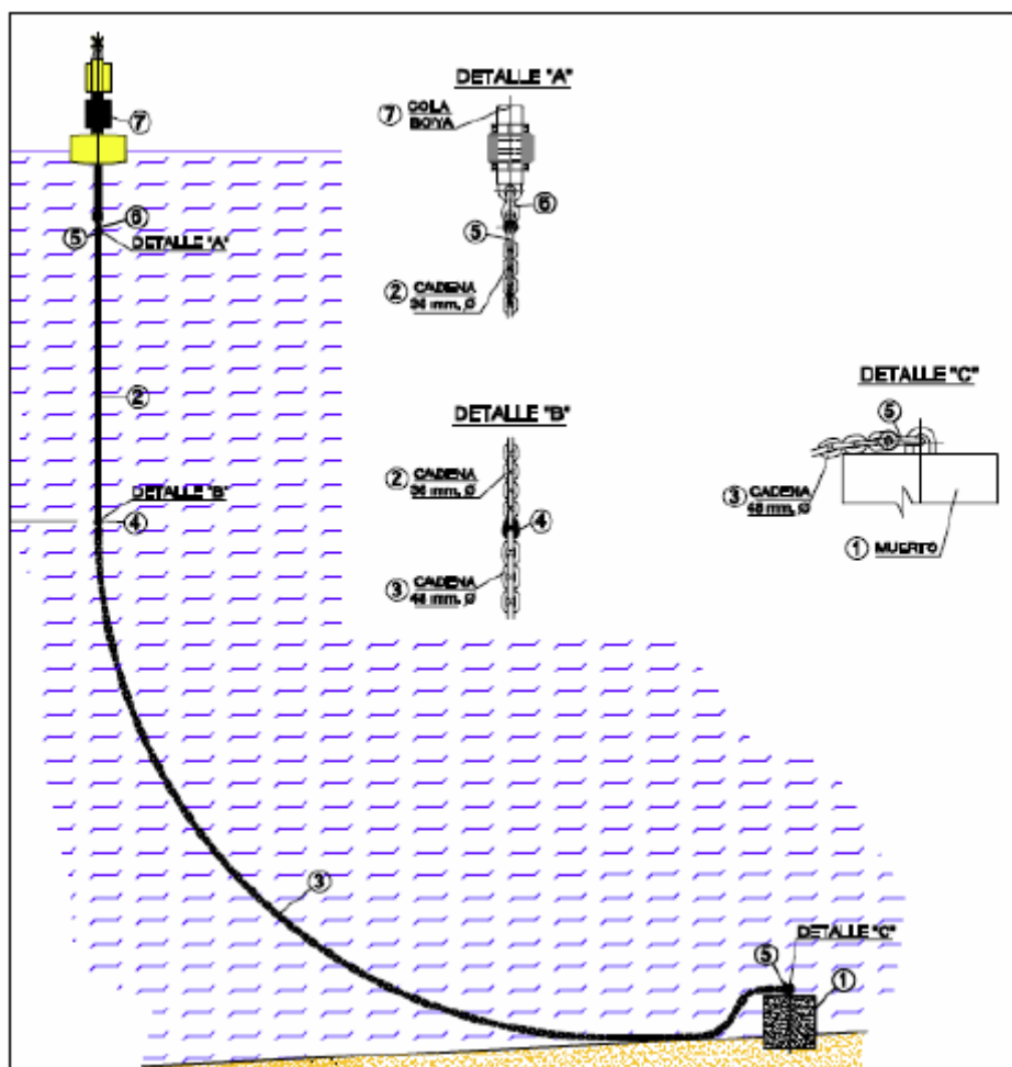
Figura 3 Tren de fondeo
