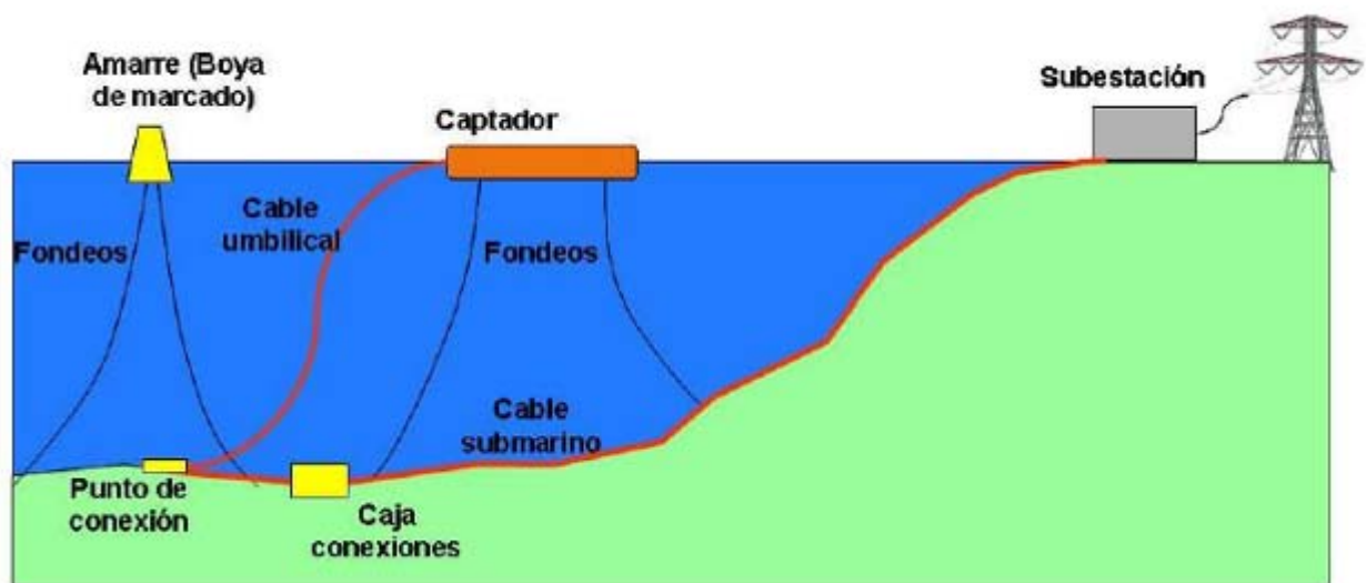
Figura 1. Esquema básico bimep - Alzado
