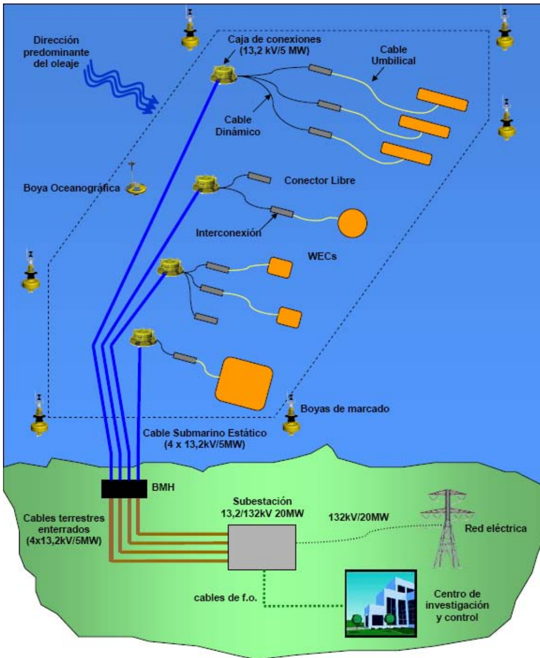
Figura 2. Esquema básico bimep - Planta
