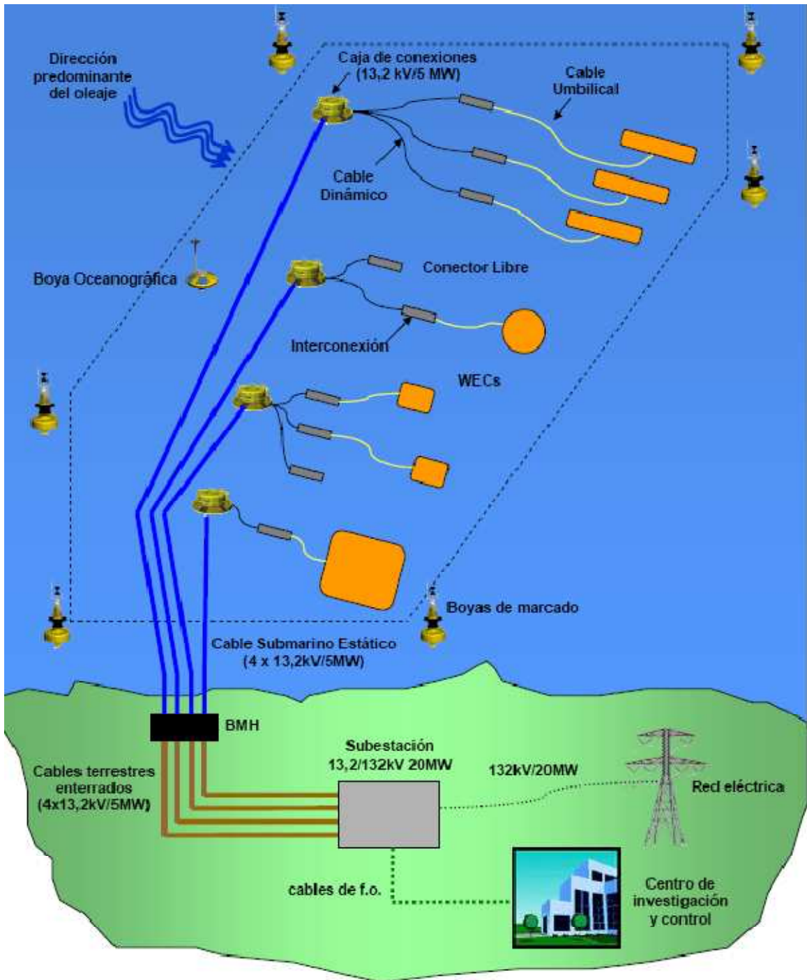
Figura 2 Esquema básico bimep - Planta
