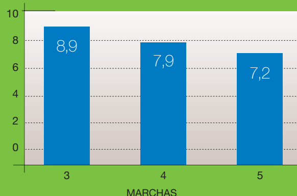
Consumo a 60 km/h (en l/100 km) - cilindrada de 2,5 l
